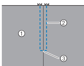
1 Лицевая сторона материала 2 Строчка 3 Конец раскрытия молнии
