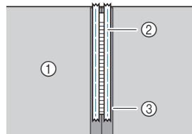
1 Изнаночная сторона материала 2 Наметочная строчка 3 Молния
